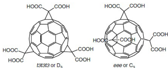
Figura 14 – Carboxifulerenos (fulerenos carboxilados) Fonte: Ros, 2008
