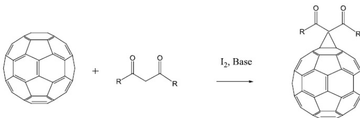
Figura 10 – Reação de adição de Ciclopropanação ao fullereno C60 Fonte: Rodrigues, 2011
