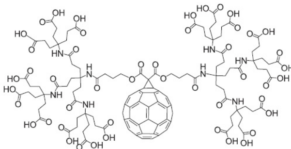
Figura 16 – Dendrofulereno, candidato ao tratamento do HIV Fonte: Santos et al. 2010
